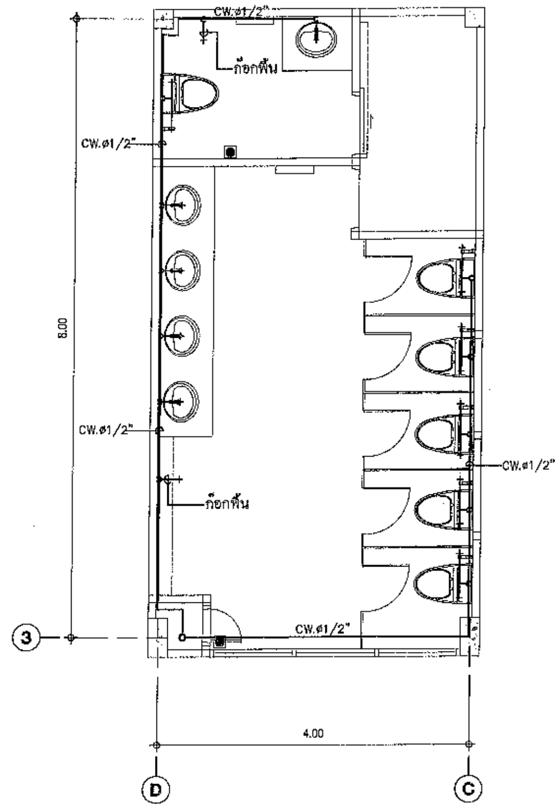
แปลนท่อน้ำดื่ม ชั้น 2 SCALE 1:75
