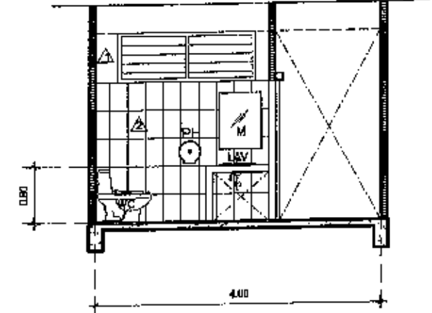
รูปตัด B SCALE 1:75
