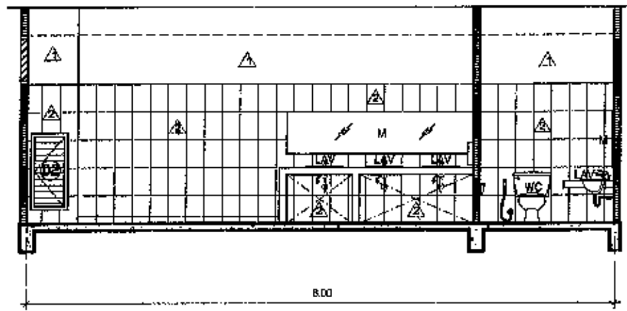
รูปตัด A SCALE 1:75
