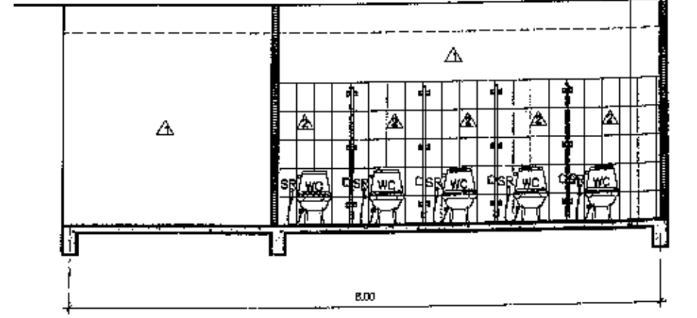
รูปตัด D SCALE 1:75
