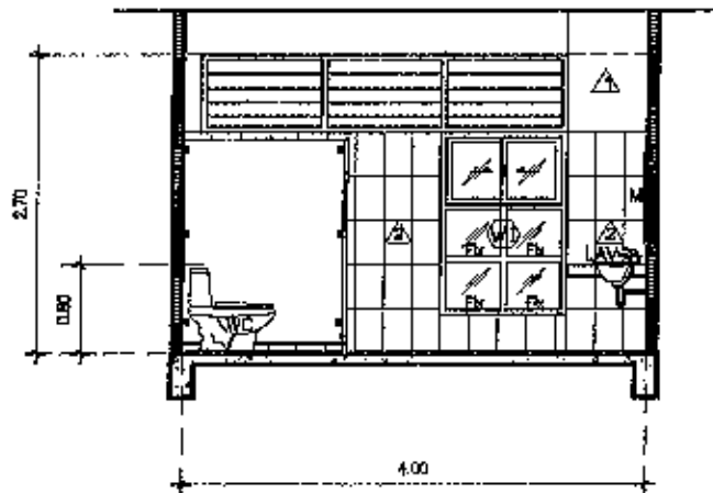
รูปตัด C SCALE 1:75
