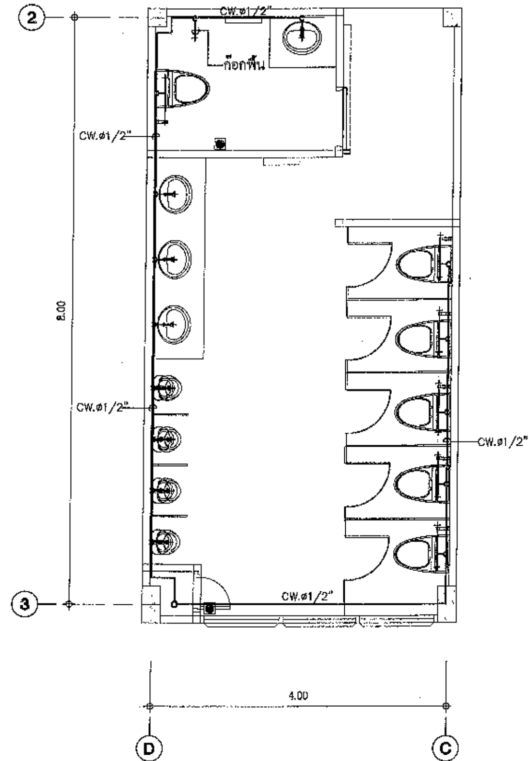
แปลนท่อน้ำดี SCALE 1:75
