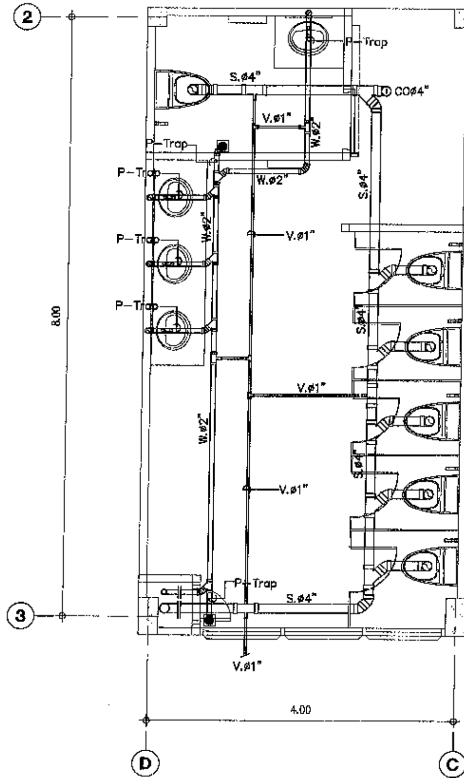
แปลนท่อน้ำทิ้ง SCALE 1:75
