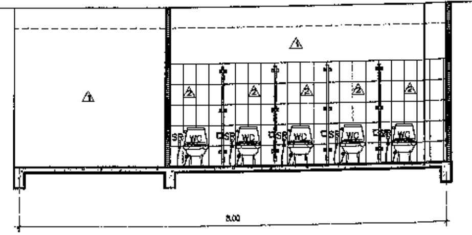
รูปตัด D SCALE 1:75
