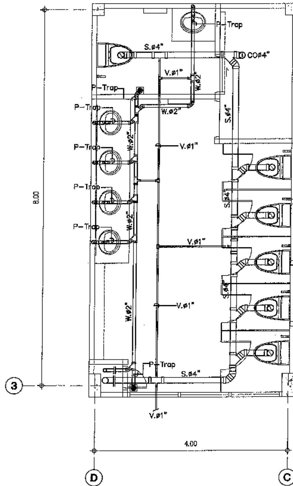
แปลนท่อน้ำทิ้ง ชั้น 2 SCALE 1:75
